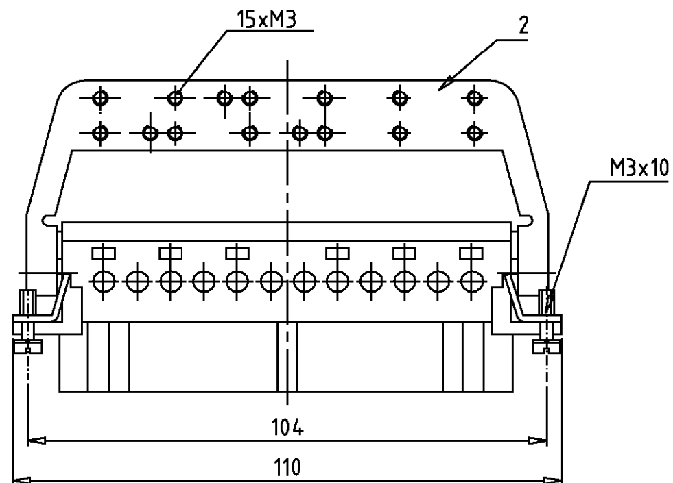
Kontaktanordnung Ansicht Anschlußseite Contact arrangement view from termination side
