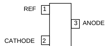
LM4041_ADJF....(SOT23)
