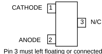
LM4041_F (SOT23)
