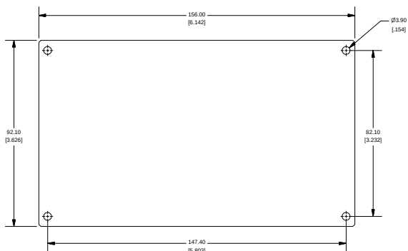
ENCLOSURE LID
