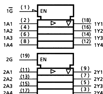
TC74HC241A
