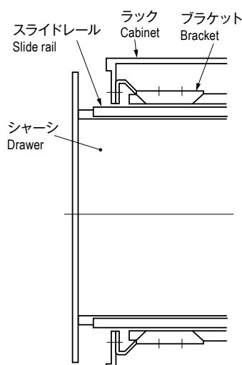
TM-169-3 取付例 Installation Example
