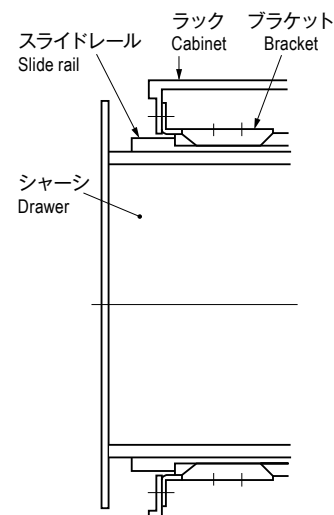
TM-169-1/TM-169-2 取付例 Installation Example
