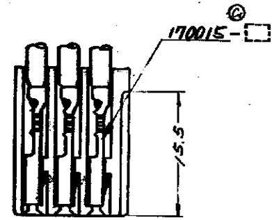
断面 A-A
