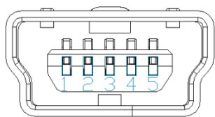
Figure 11: Mini USB Connector
