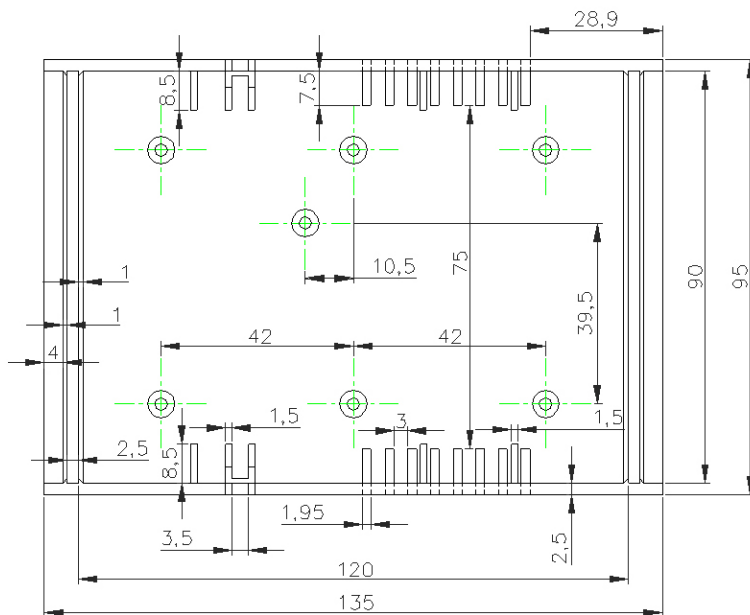
Gehäuseober- bzw. unterteil
