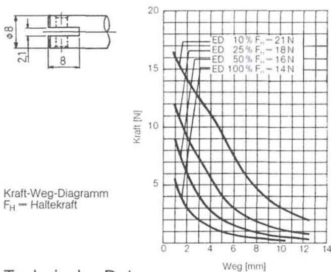
Ankerdetail
