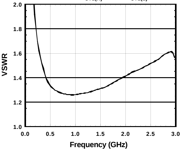
VSWR(P4) vs. Frequency
