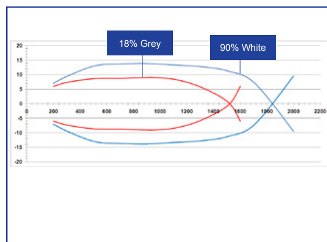
Background suppression
