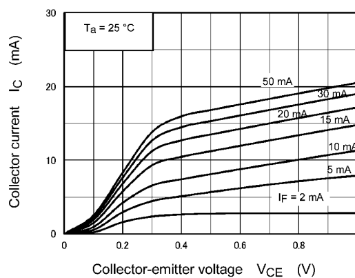
Fig. 11.8 I_C - V_{CE}
