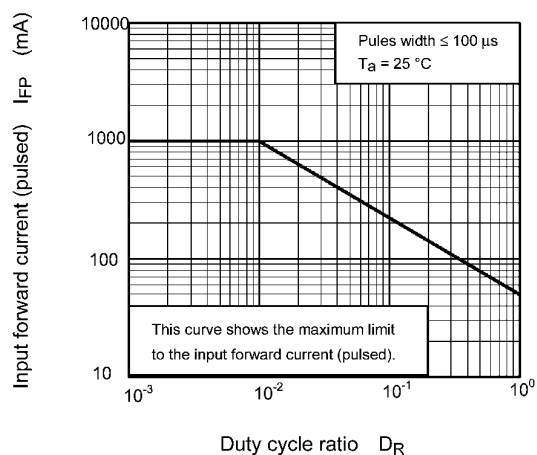
Fig. 11.3 I_{FP} - D_R
