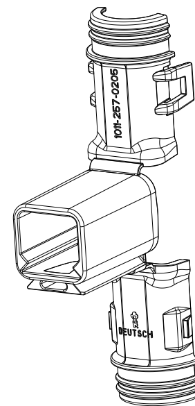
SCALE 1:1 Maßstab
