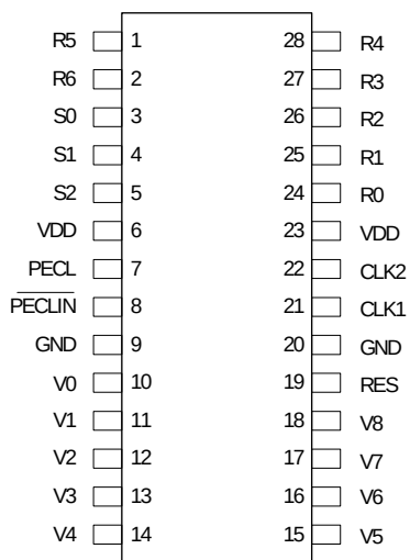
28-pin SSOP
