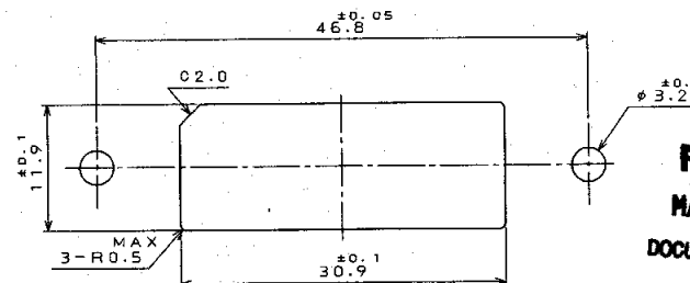
MOUNTING PANEL CUTOUT DIMENSIONS (REF.) パネル取付寸法 (参考)
