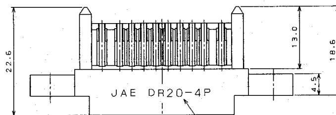
JAE AND PART NO. MARKING 社標及び品名表示
