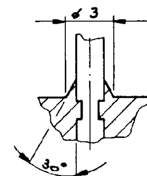
EINZELHEIT Y M 5:1
