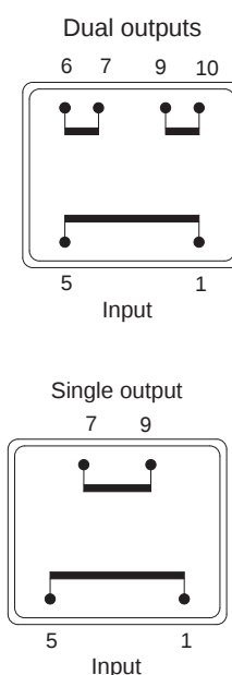
WIRING DIAGRAM:
