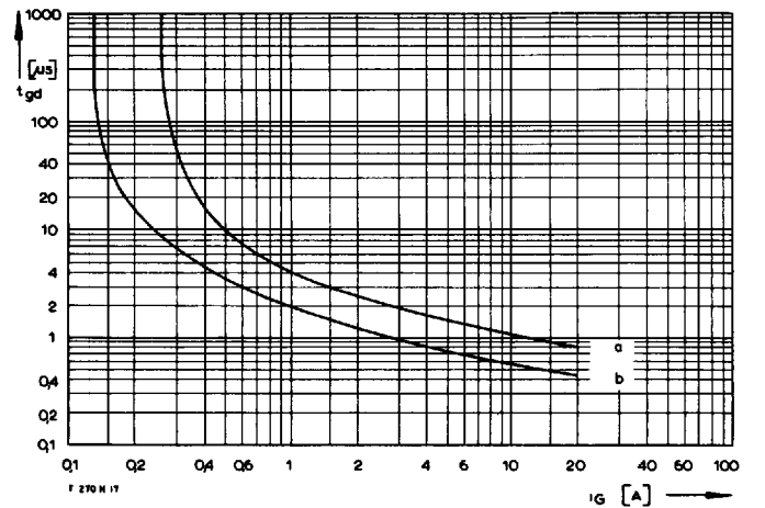
Bild/ Fig. 18 Zündverzögerung t_{gd} bei I_{TM} = 100 \text{ A} , t_{vj} = 25^\circ\text{C} . Gate controlled delay time t_{gd} at I_{TM} = 100 \text{ A} , t_{vj} = 25^\circ\text{C} . a – äußerster Verlauf/limiting characteristic b – typischer Verlauf/typical characteristic
