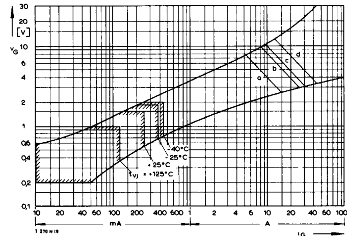
Bild/ Fig. 17 Zündbereich und Spitzensteuerleistung bei v_D \geq 6 \text{ V} . Gate characteristic and peak gate power dissipation at v_D \geq 6 \text{ V} . Parameter: Steuerimpulsdauer/Pulse duration t_g [ms] a b c d Höchstzulässige Spitzensteuerleistung/ Maximum allowable peak gate power [W] 40 80 100 150
