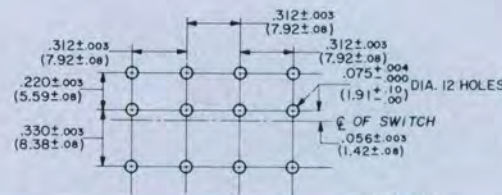
P.C. LAYOUT
