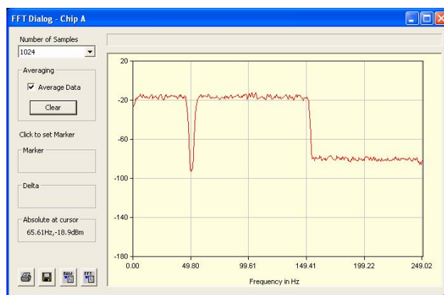
Actual Filter Output from QF1D512
