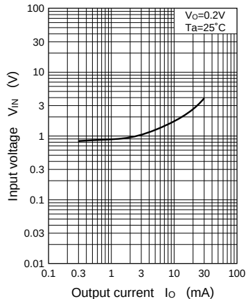
V_{IN} - I_O
