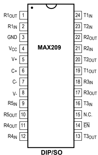
DIP/SO
