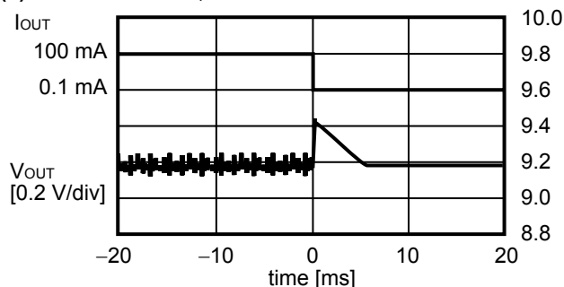
(4) f_{OSC} = 700\text{ kHz} , I_{OUT} = 100\text{ mA} \rightarrow 0.1\text{ mA}
