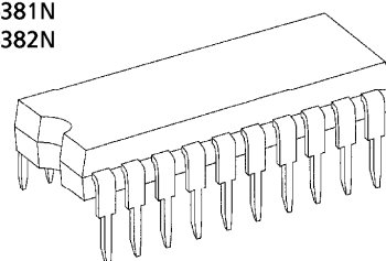
SDIP20-P-300-1.78
