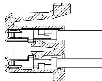
ターミナル装着図 TERMINAL ASSEMBLY DRAWING
