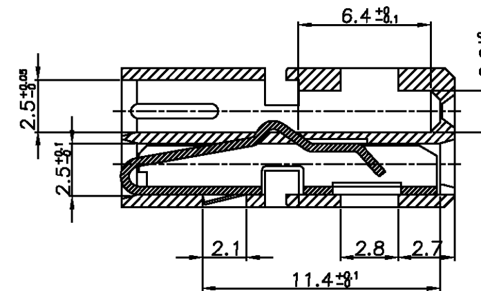
SECT A-A
