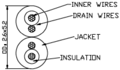
CABLE SEC(A-A')
