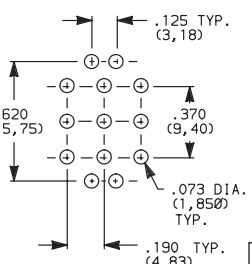
7301J1_BE2 3PDT
