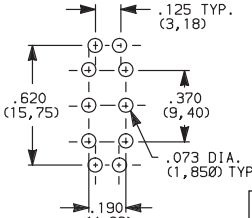
7201J1_BE2 DPDT
