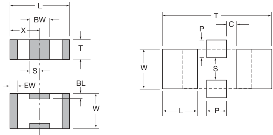
W2H1 - 0805 Style
