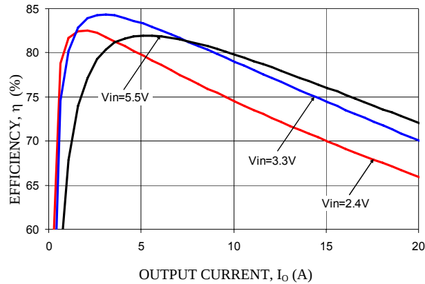
V_o=0.6V
