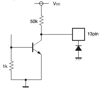
Bias-drop mute
