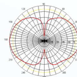
E-plane-vertical
