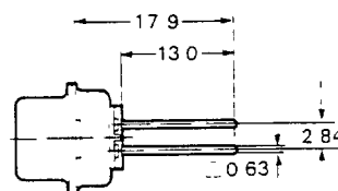
Wire Wrap
