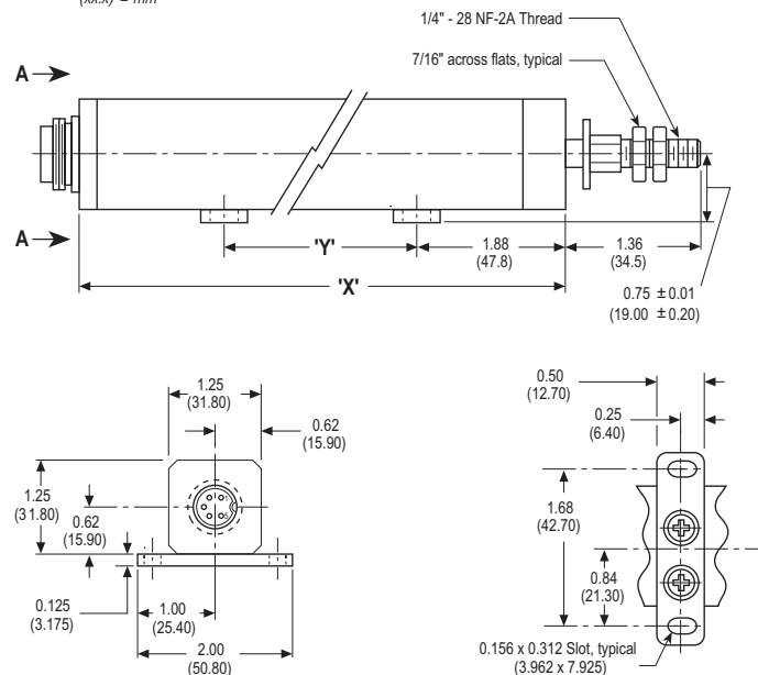
VIEW A-A
