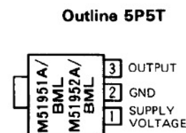
Outline SOT-89
