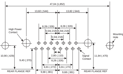
B 17W2 15 #20 2 #8
