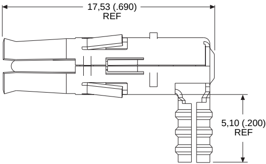
Receptacle
