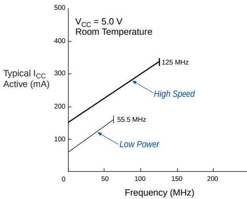
EPM7128E
