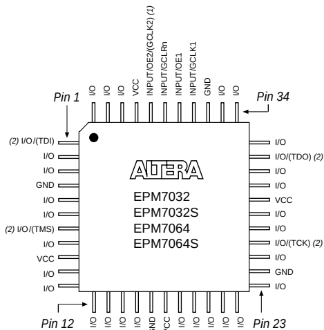
44-Pin TQFP
