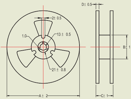
Reel Dimensions
