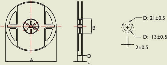
Reel Dimensions
