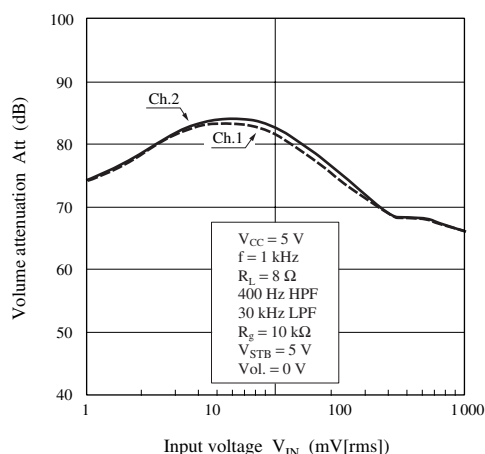
Att — V_{IN}
