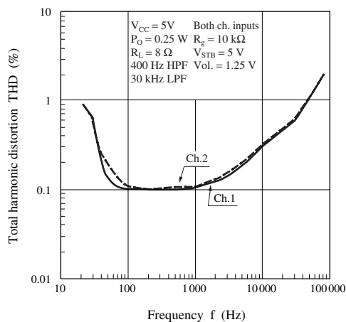
THD — f
