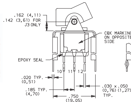
7401J1_BE2 4PDT
