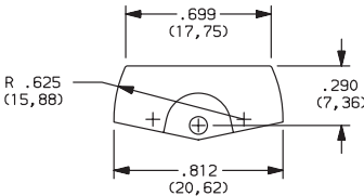
J8 ROCKER
