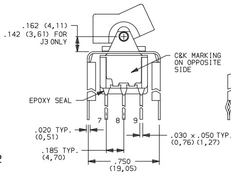
7301J1_BE2 3PDT
