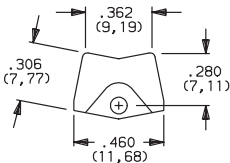
J50 ROCKER
