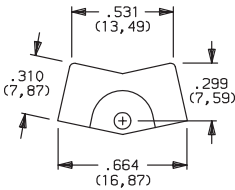
J1 ROCKER
