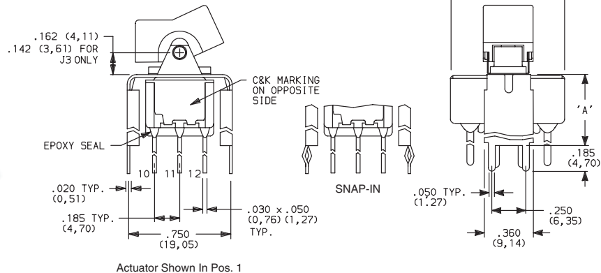
7401J1_BE2 4PDT
