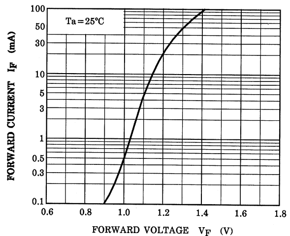
I_F - V_F
