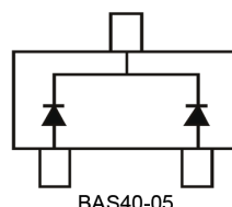
BAS40-05
