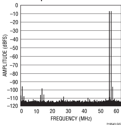
LTC2195: 64k Point 2-Tone FFT, f_{IN} = 69\text{MHz} , 70\text{MHz} , -7\text{dBFS} , 125\text{Mps}
