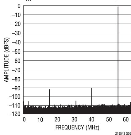
LTC2195: 64k Point FFT, f_{IN} = 70\text{MHz} , -1\text{dBFS} , 125\text{Mps}
