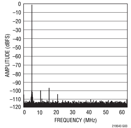
LTC2195: 64k Point FFT, f_{IN} = 5\text{MHz} , -1\text{dBFS} , 125\text{Mps}
