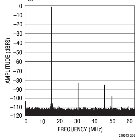
LTC2195: 64k Point FFT, f_{IN} = 140\text{MHz} , -1\text{dBFS} , 125\text{Mps}
