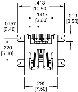
MUSB-10P-S-RA-M1-SMT
