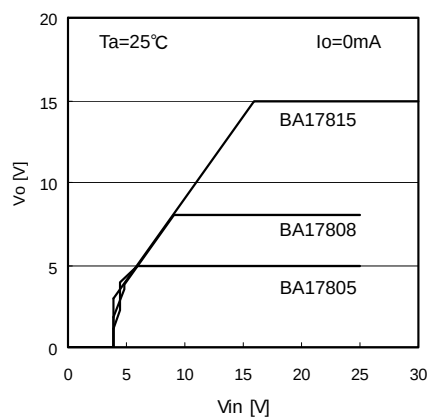
Fig.13 電源電圧－出力電圧 ( I_o=0\text{mA} )
