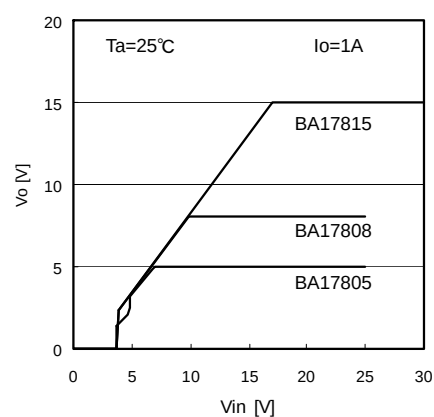
Fig.15 電源電圧－出力電圧 ( I_o=1\text{A} )
