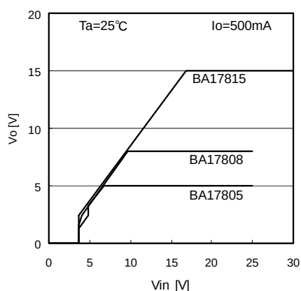
Fig.14 電源電圧－出力電圧 ( I_o=500\text{mA} )
