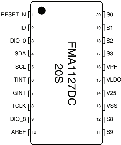
20-Pin SSOP
