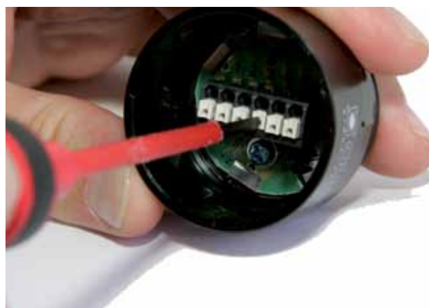
Anschlussklemme mit Push-In Technik (ECModul40)
