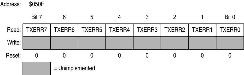
Figure 21-25. Transmit Error Counter (CTXERR)
