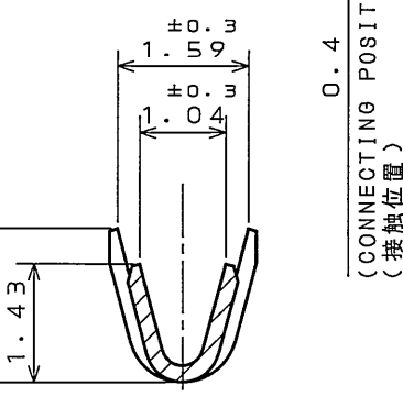
SECTION A-A (断面 A-A)
